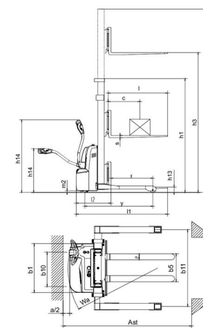
CTD12R-E
