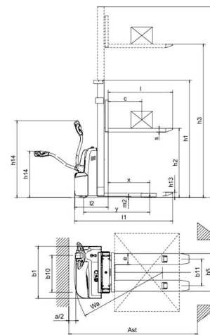
CDD10R-E/CDD12R-E/CDD15R-E
